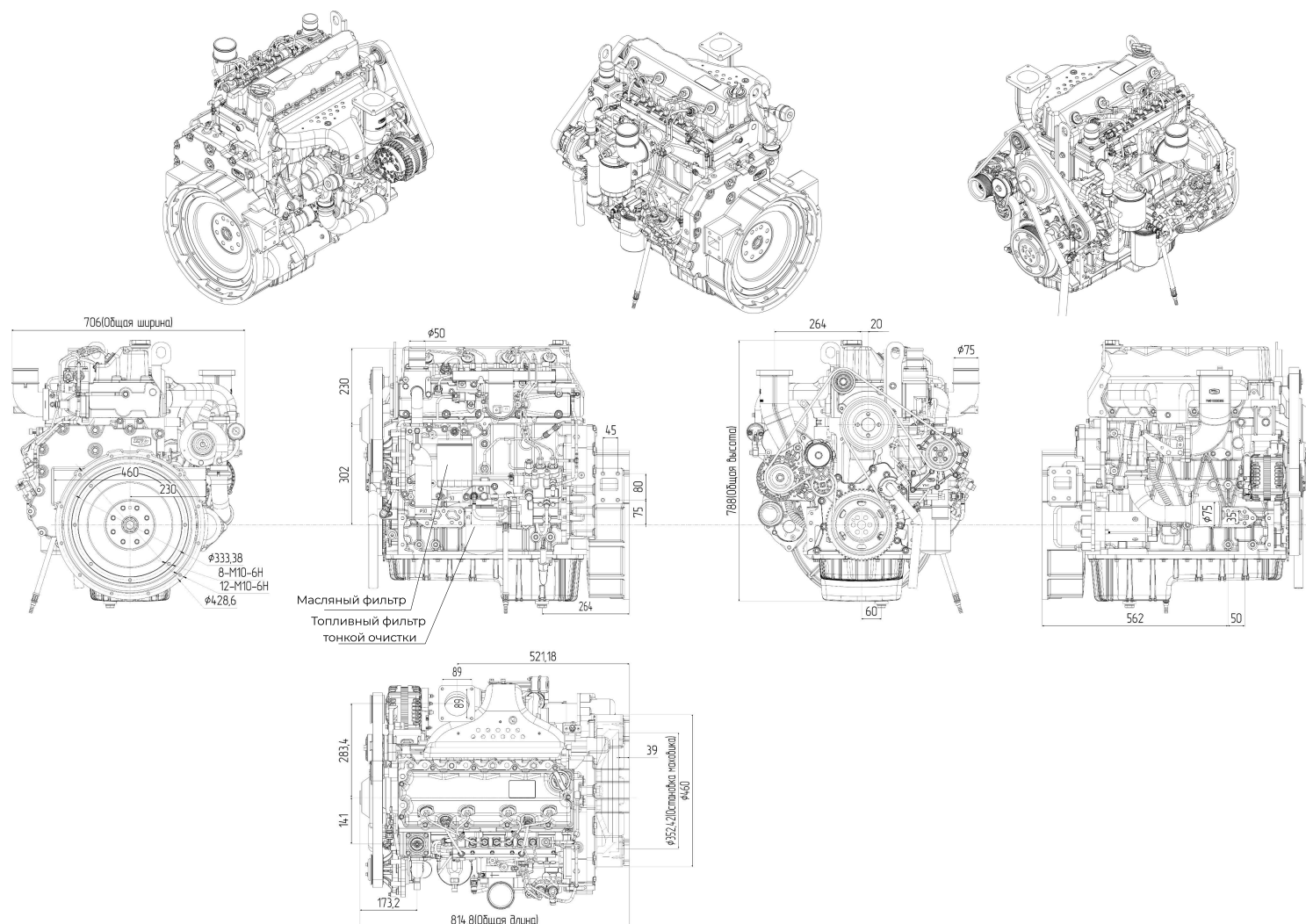
Схема двигателя DEF47CTD4
